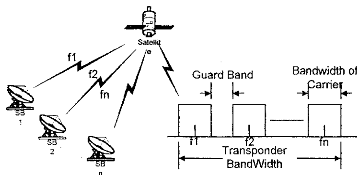
Gambar 3. Sistem Transmisi FDMA
