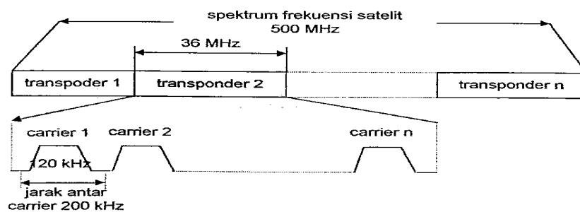
Gambar 2. Spektrum Frekuensi Satelite
